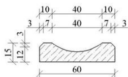
WIDOK Z GÓRY
