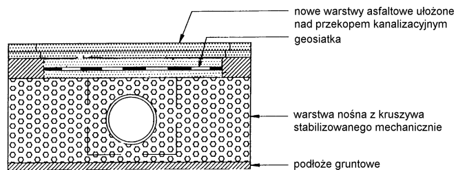
Rys. 1. Wzmocnienie nawierzchni asfaltowej nad przekopem instalacyjnym
