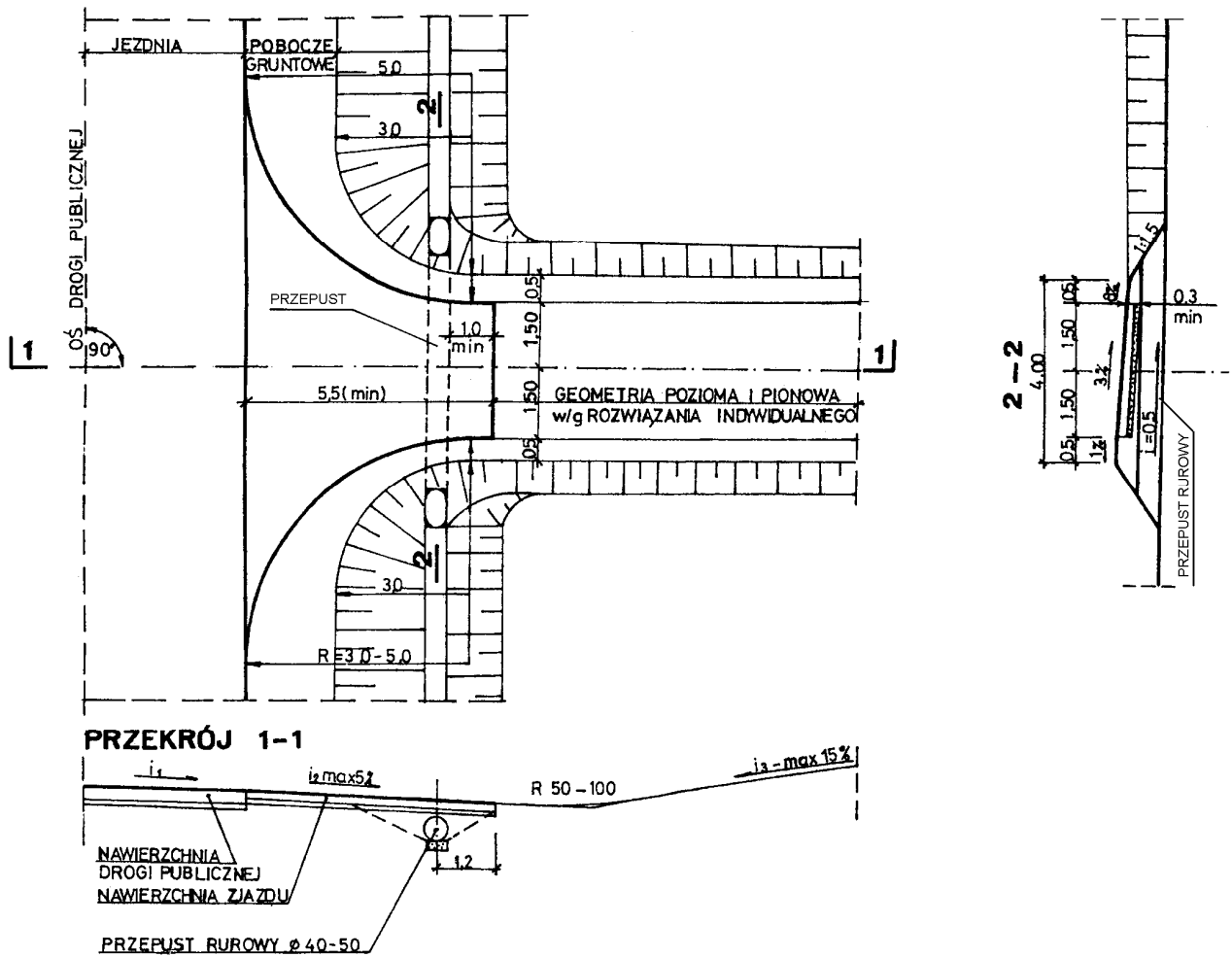
Rys. 3.1. Przykładowe rozwiązanie sytuacji zjazdu indywidualnego z przepustem
