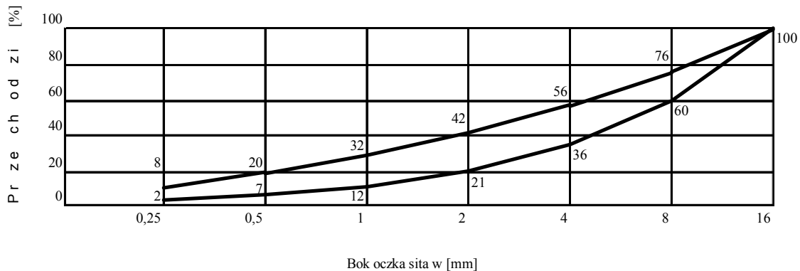
Krzywa uziarnienia kruszyw 0 - 16 mm
