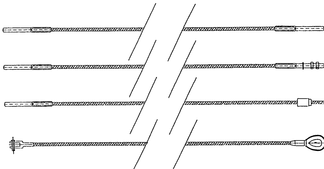
Rys. 7. Przykłady lin stalowych stosowanych w barierach linowych
