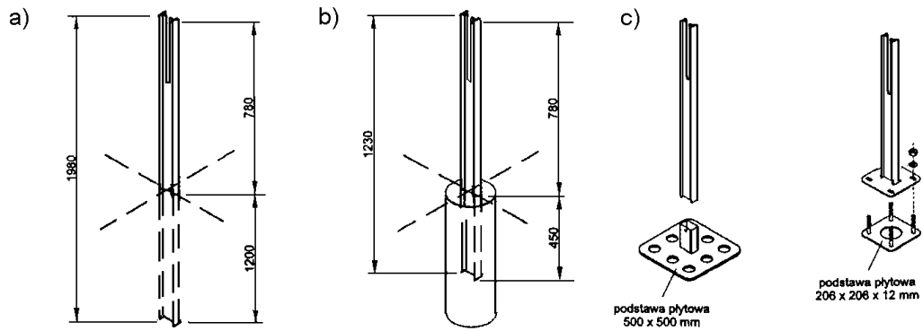
Rys. 6. Przykłady ukośnego odcinka początkowego bariery linowej
