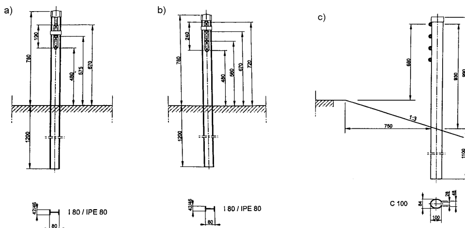
Rys. 4. Przykłady ustawienia słupków barier linowych a) Bariera trzylinowa skrajna lub dzieląca, b) Bariera czterolinowa skrajna lub dzieląca, c) Bariera czterolinowa skarpowa
