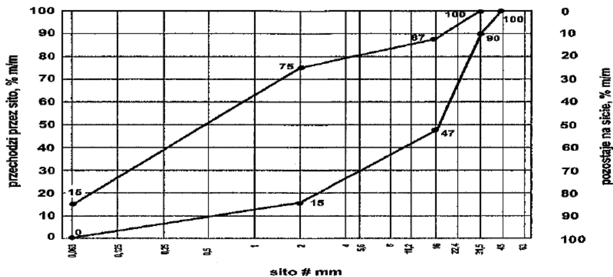
Wykres 1 Wymagania uziarnienia stawiane warstwie kruszywa 0/31.5
