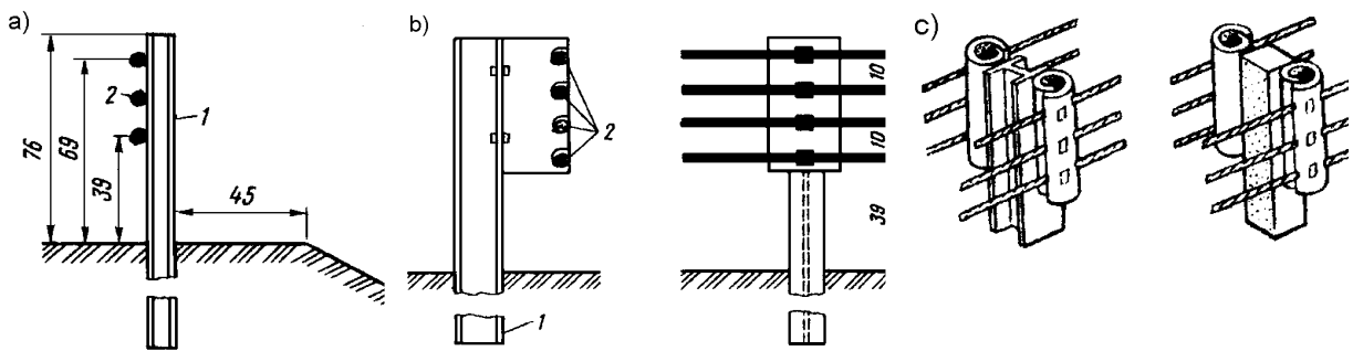
Rys. 4. Przykłady ustawienia słupków barier linowych a) Bariera trzylinowa skrajna lub dzieląca, b) Bariera czterolinowa skrajna lub dzieląca, c) Bariera czterolinowa skarpowa
