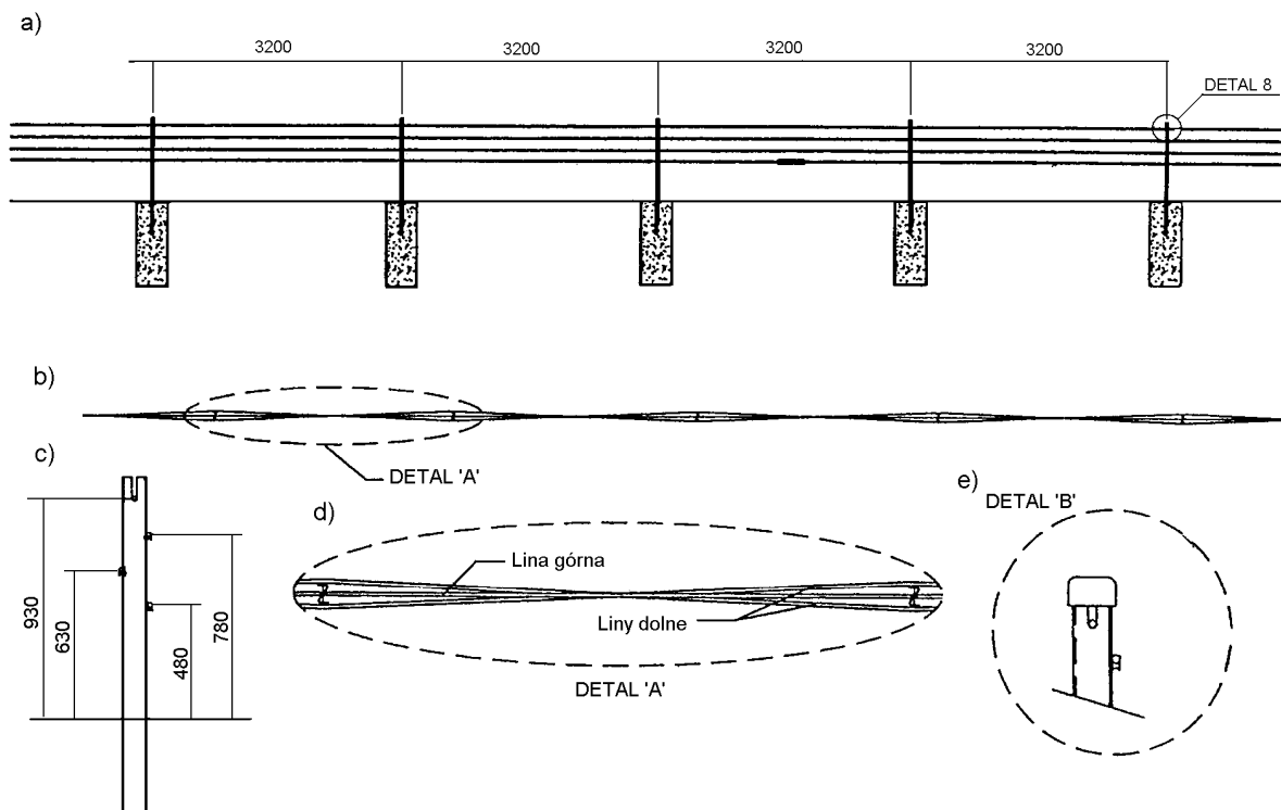
Rys. 9. Przykładowy schemat bariery czterolinowej
