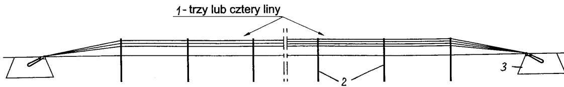
Rys. 3. Przykłady umocnienia lin do słupków a) Bariera trzylinowa, b) Bariera czterolinowa, c) Bariera trzylinowa dwustronna na słupku dwuteowym i prostokątnym, 1 – słupek, 2 – lina
