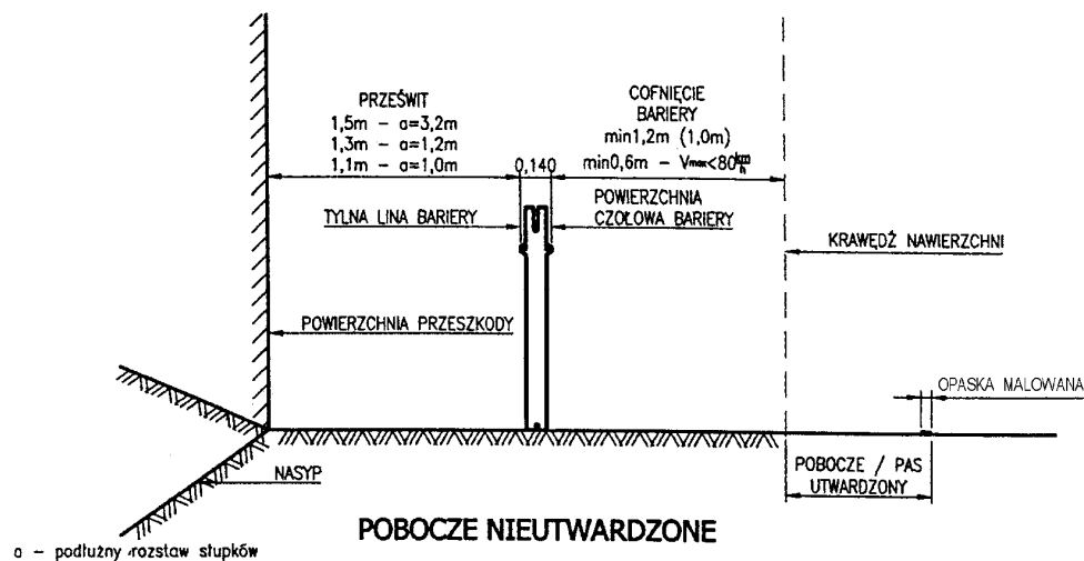
Rys. 1.2. Lokalizacja bariery linowej w pasie dzielącym drogi dwujezdniowej
