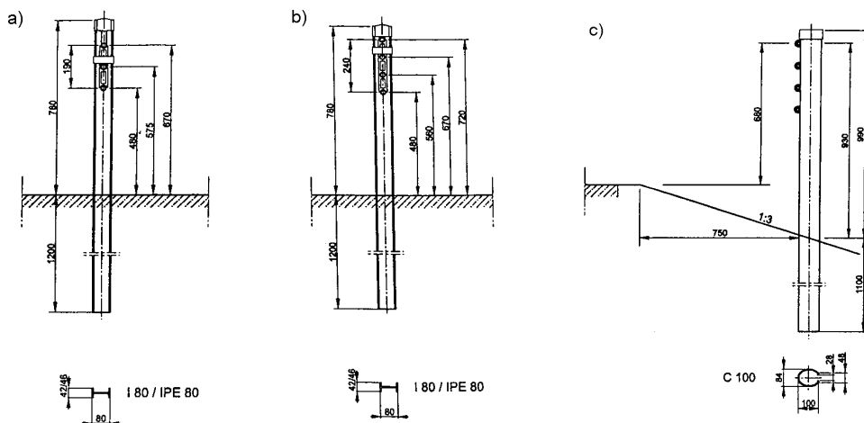
Rys. 5. Sposoby osadzenia w gruncie i przymocowania słupków barier linowych a) Słupek zagłębiony w gruncie, b) Słupek osadzony w fundamencie betonowym, c) Słupki z metalową podstawą płytową do przymocowania na obiekcie mostowym
