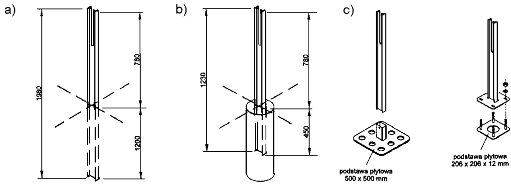
Rys. 6. Przykłady ukośnego odcinka początkowego bariery linowej
